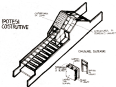
Casa a schiera: autocostruzione parziale. Ipotesi tecnologica. Le possibili modalità di crescita nel tempo. Da: AA.VV. (1985), Costruzione facilitata. Milano: BE-MA, p. 20.
